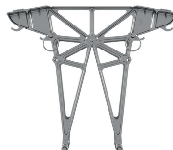
Mittlere Stütze 15° für Süd Ausrichtung
